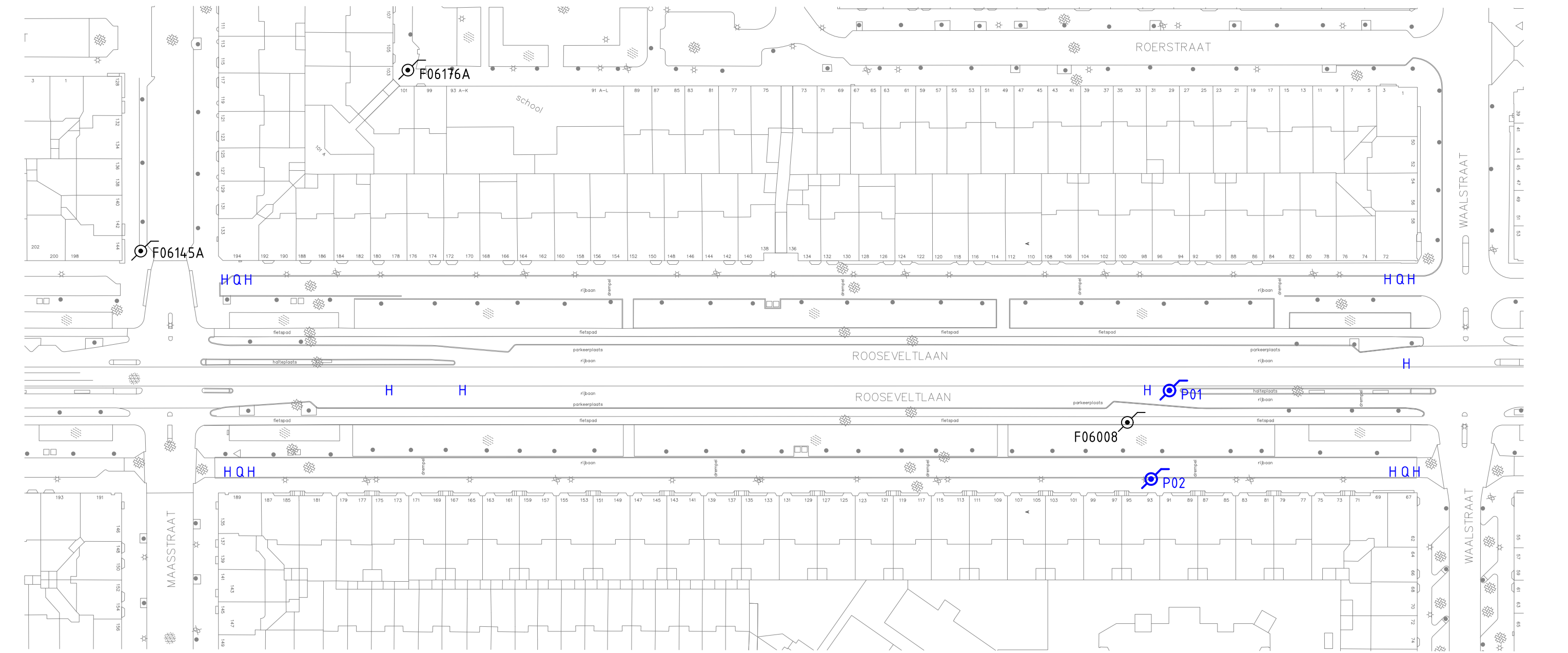
Situatie peilbuizen en meetpunten Schaal 1:1000
